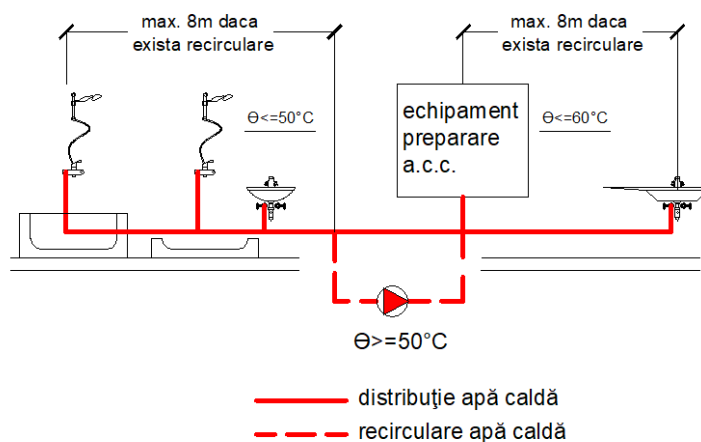
Figura 11.3. Preparare individuală a apei calde, cu recirculare (traseul de distribuție este mai lung de 30 m), temperatura apei calde se va menține la minim 50^{\circ}\text{C} .
