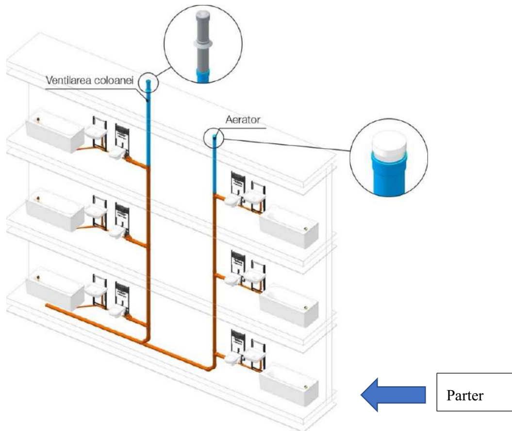
Figura A5.9.2 - Exemplu de ventilare principală, cu aerator cu membrană, pentru o clădire cu maxim 3 niveluri, dotată cu obiecte sanitare; obiectele sanitare de la parter sunt racordate la coloana de canalizare. Aeratorul poate fi montat pentru coloane la care nu sunt racordate mai mult de 9 obiecte sanitare.
