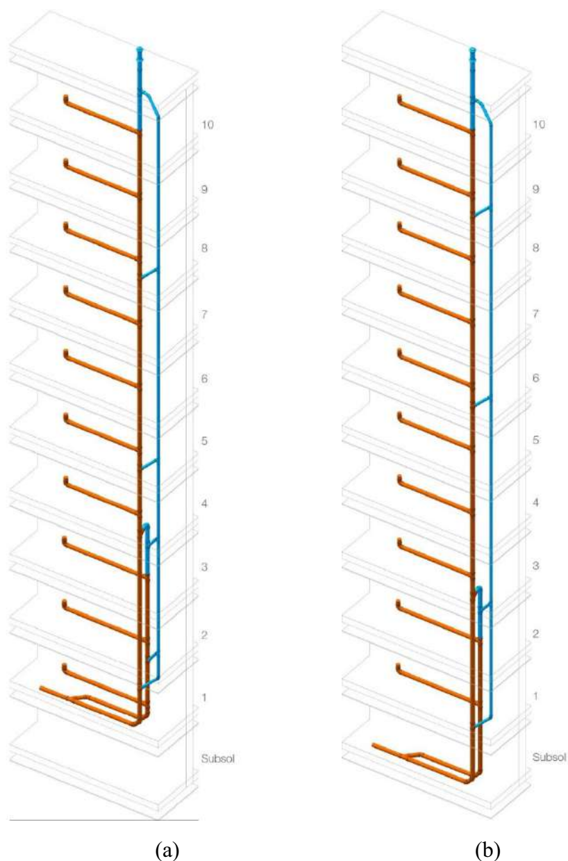
Figura A5.9.13– Exemple de ventilare primară și auxiliară, aplicate unei instalații de canalizare, pentru o clădire cu peste 10 niveluri; dotarea cu ventilare auxiliară se realizează în condițiile descrise în capitolul 13.
