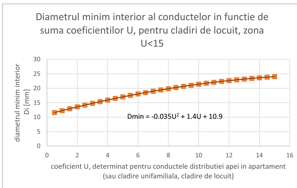
Figura 11.1- metoda de determinare directă a diametrului minim al conductelor amplasate în interiorul clădirilor de locuit, pentru U < 15 .
