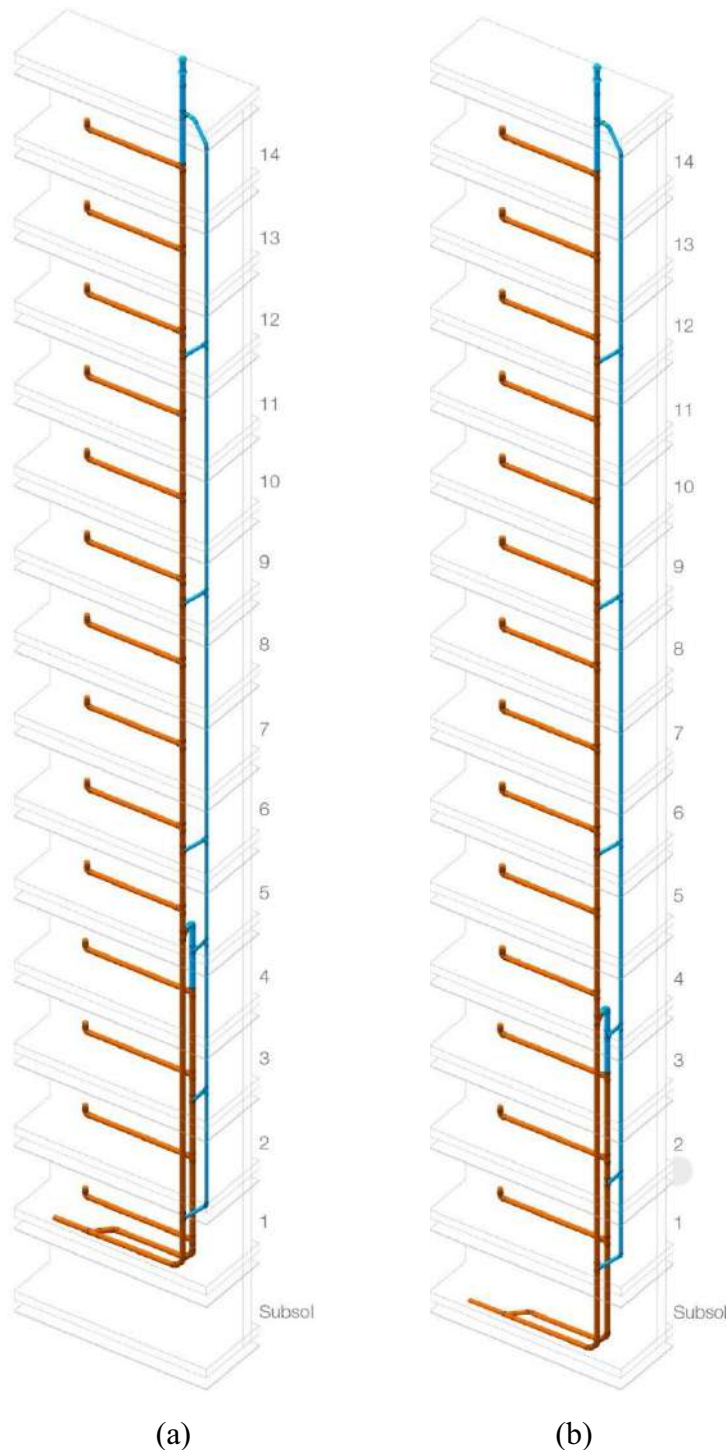
Figura A 5.9.14– Exemple de ventilare primară și auxiliară, aplicate unei instalații de canalizare, pentru o clădire cu peste 14 niveluri; dotarea cu ventilare auxiliară se realizează în condițiile descrise în capitolul 13.
