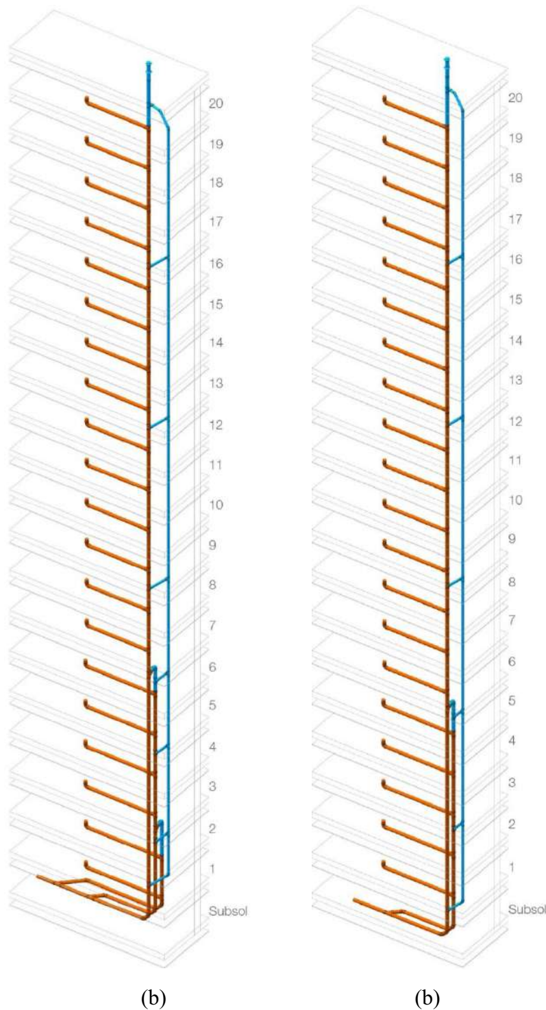
Figura A 5.9.15– Exemple de ventilare primară și auxiliară, aplicate unei instalații de canalizare, pentru o clădire cu peste 20 niveluri; dotarea cu ventilare auxiliara se realizează în condițiile descrise în capitolul 13.
