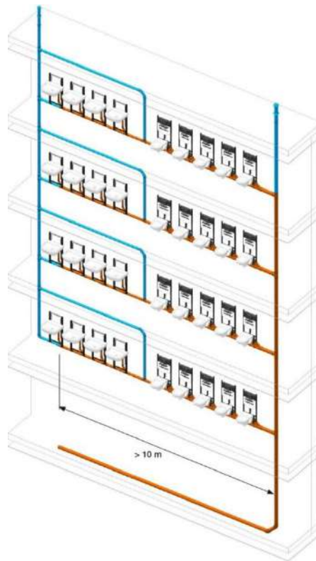
Figura A5.9.12 – Exemple de ventilare primară și secundară, aplicate unei instalații de canalizare, cu conducte de legătură cu lungimi peste 10 m, pentru care se adoptă ventilare secundară; pentru conducte de legătură cu lungimi peste 10 m, se recomandă introducerea unei conducte de ventilare secundară intermediară pe traseul conductelor de legătură.
