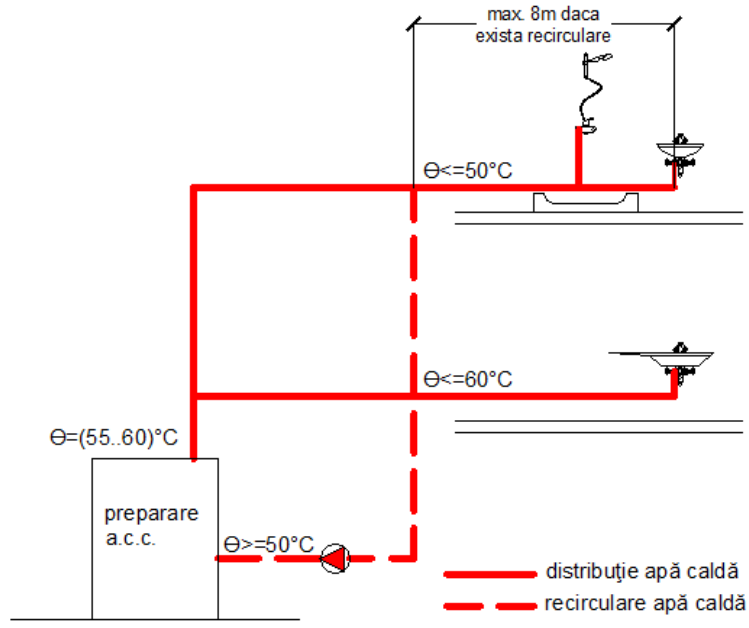
Figura 11.1 Preparare centralizată a apei calde, lungimea maximă a racordurilor / conductelor de legătură este de 8m, în situația în care s-a prevăzut recirculare.
