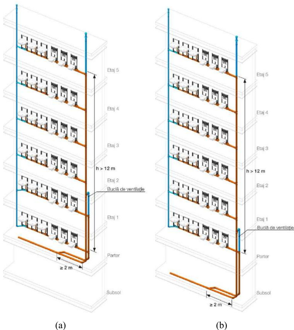
Figura A 5.9.11 (a), (b) – Variante suplimentare de ventilație secundară, pentru clădiri cu peste 5 niveluri, pentru care h > 12\text{ m} . Dotarea cu ventilație secundară se realizează în condițiile descrise în capitolul 13.
